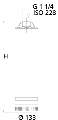
Рис. 2: Насос Ixo N
