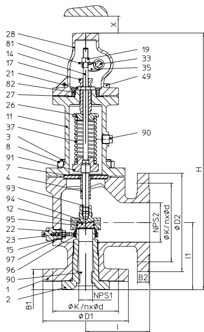
Фиг. ... 971 Устройство для принудительного открытия в закрытом исполнении
