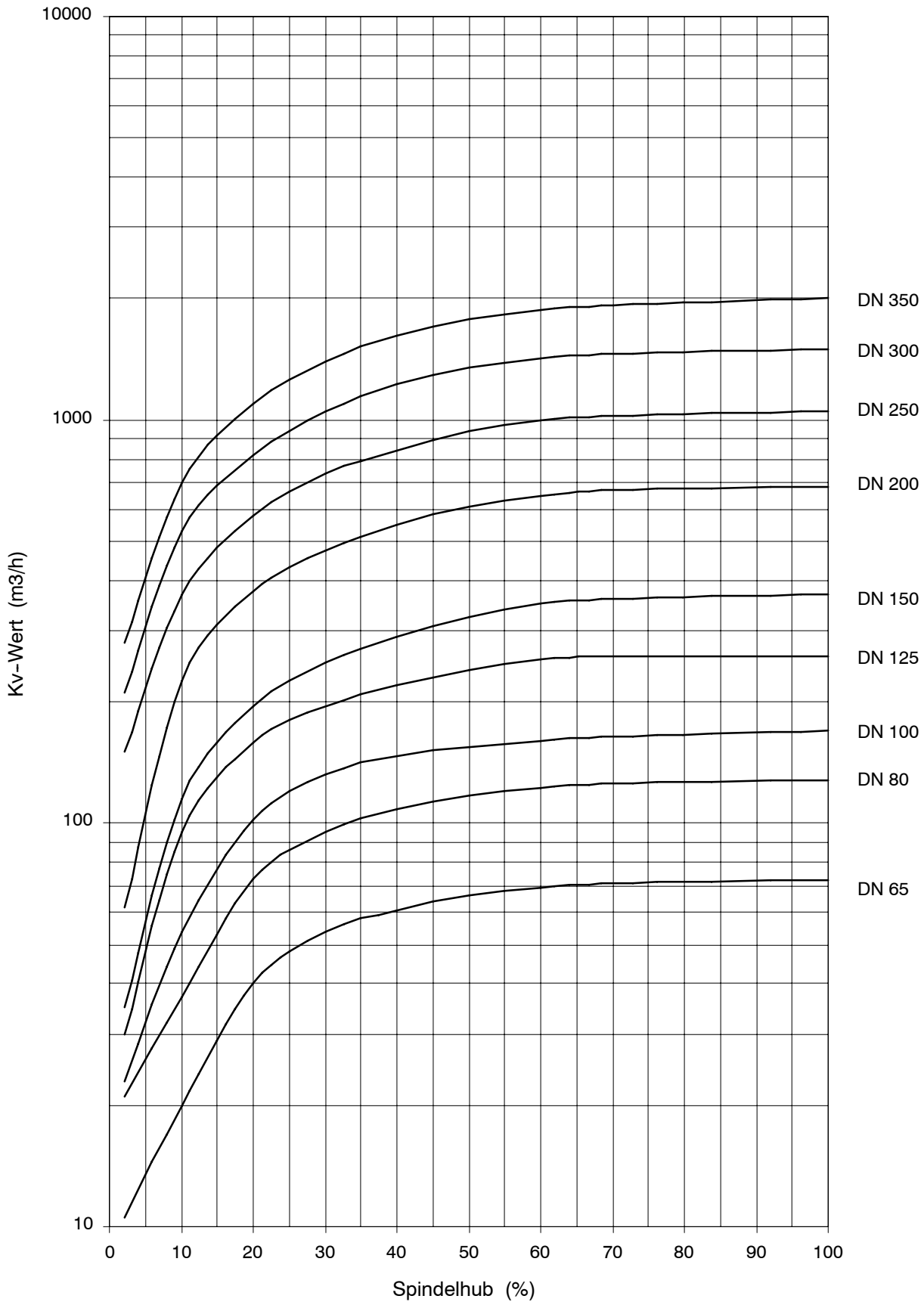
K_v - Wert in Abhängigkeit vom Spindelhub
